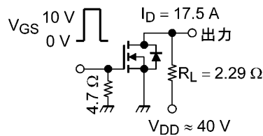
図 6.2.1 スwitchング時間の測定回路例
