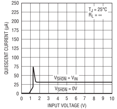
LT1763-1.5の消費電流
