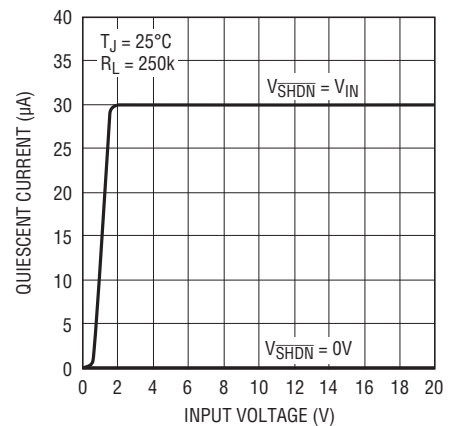
LT1763の消費電流
