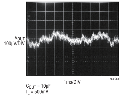
LT1763-5の 10Hz~100kHz出力ノイズ C_{BYP} = 1000\text{pF}
