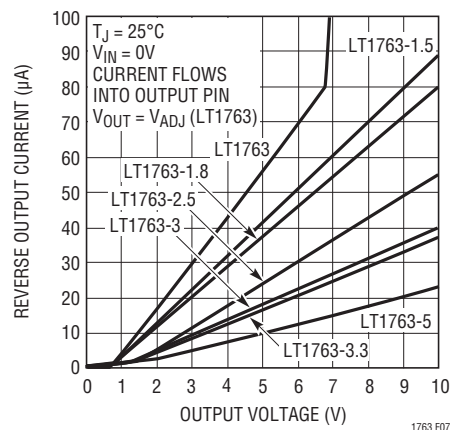
図7. 逆出力電流
