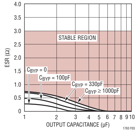
図3. 安定性
