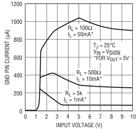
LT1763-5のGNDピン電流
