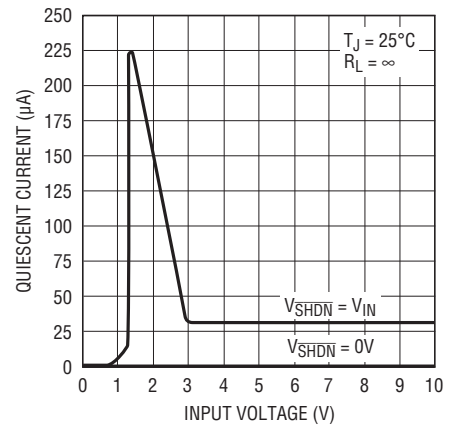
LT1763-3の消費電流
