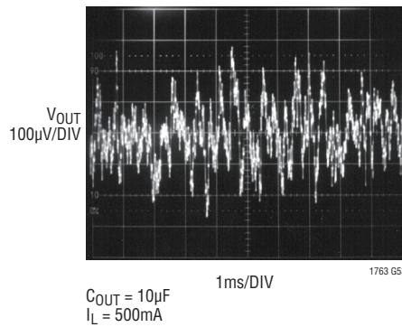
LT1763-5の 10Hz~100kHz出力ノイズ C_{BYP} = 100\text{pF}
