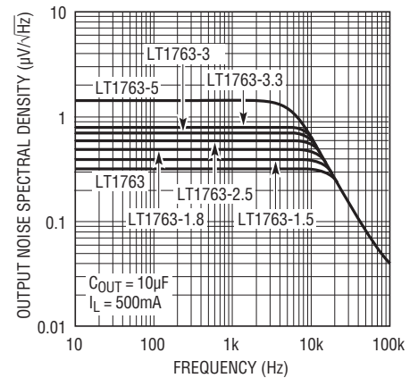
出力ノイズのスペクトル密度 C_{BYP} = 0
