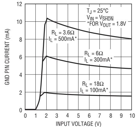
LT1763-1.8のGNDピン電流
