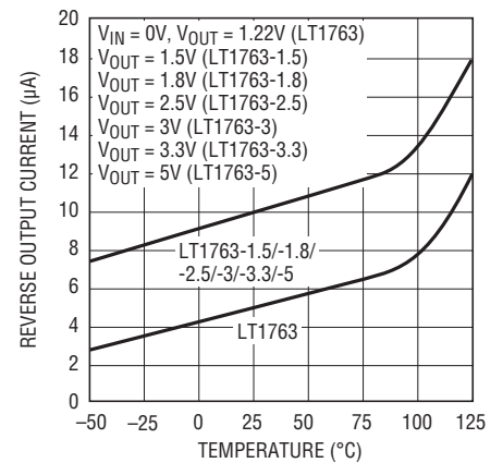
逆出力電流
