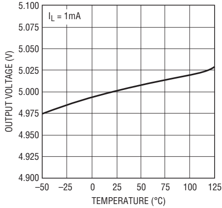
LT1763-5の出力電圧
