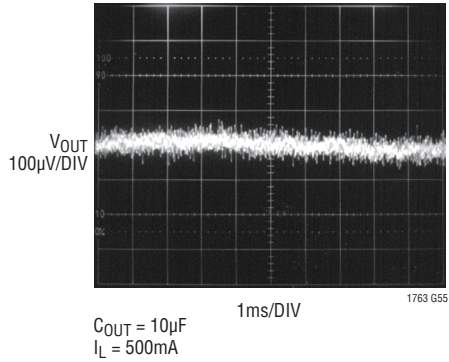
LT1763-5の 10Hz~100kHz出力ノイズ C_{BYP} = 0.01\mu F
