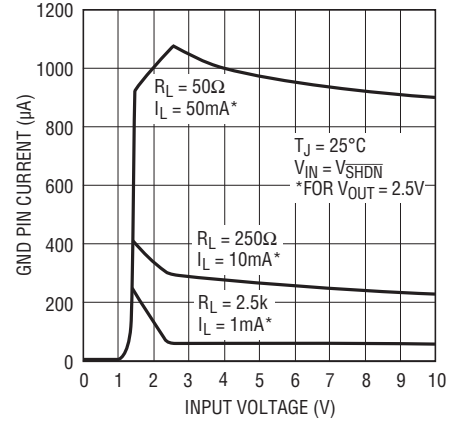
LT1763-2.5のGNDピン電流
