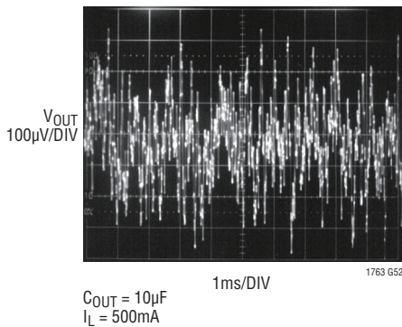
LT1763-5の 10Hz~100kHz出力ノイズ C_{BYP} = 0
