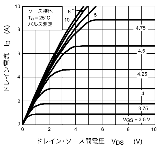
図 8.1 I_D - V_{DS}
