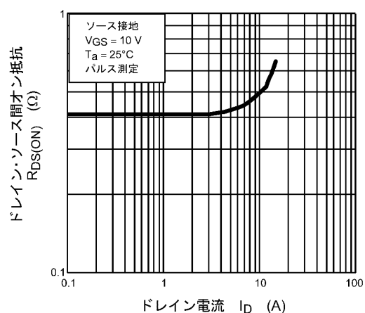
図 8.6 R_{DS(ON)} - I_D
