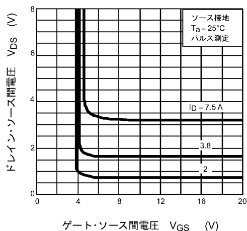
図 8.4 V_{DS} - V_{GS}
