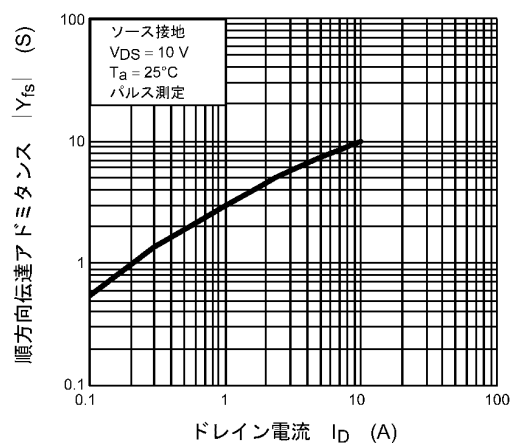
図 8.5 |Y_{fs}| - I_D
