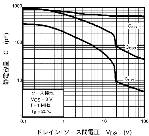
図 8.9 C - V_{DS}
