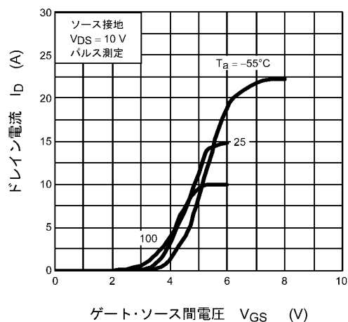
図 8.3 I_D - V_{GS}
