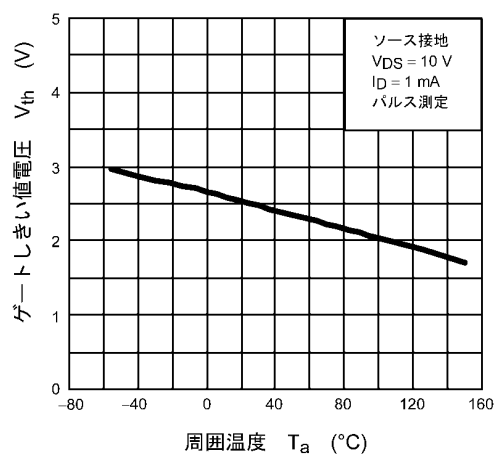
図 8.10 V_{th} - T_a
