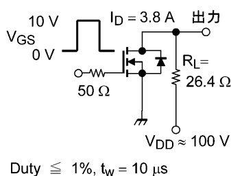
図 6.2.1 スwitchング時間の測定回路例
