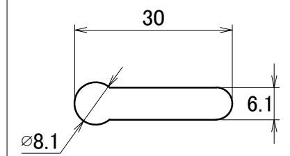
長穴詳細図
