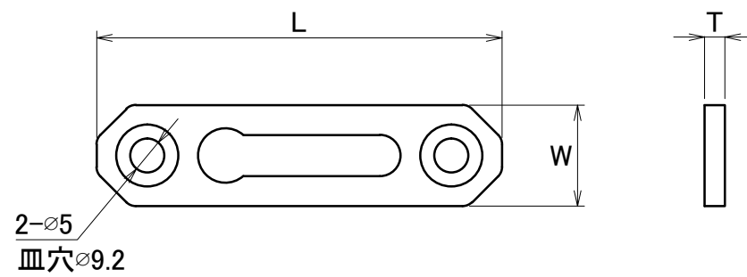
長穴詳細図
