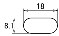
長穴詳細図
