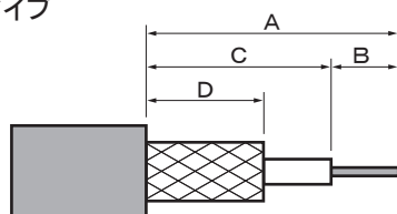
ケーブルカット寸法 同軸ケーブルタイプ
