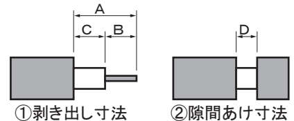
ケーブルカット寸法 セミリジットケーブルタイプ
