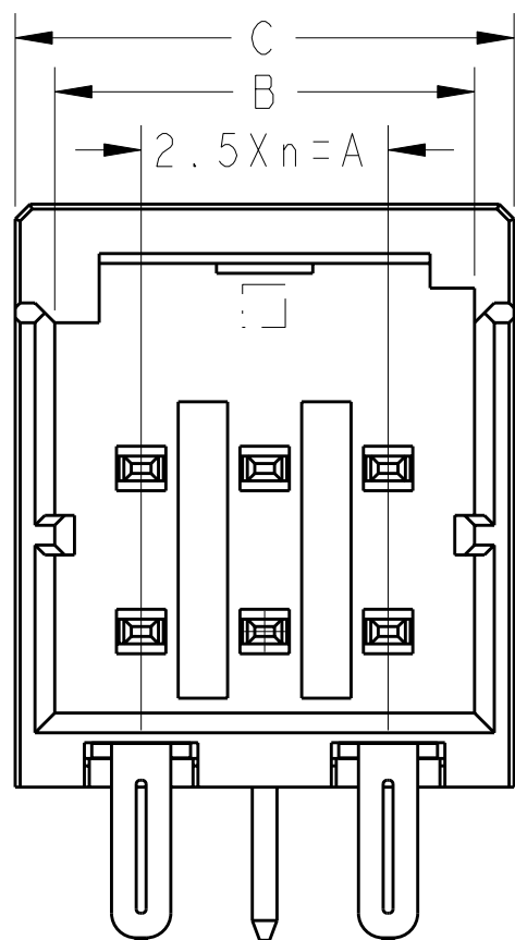
I-1827876-3 (6POS:X-KEY)
