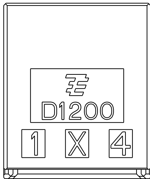
I-1827876-4 (8POS:X-KEY)
