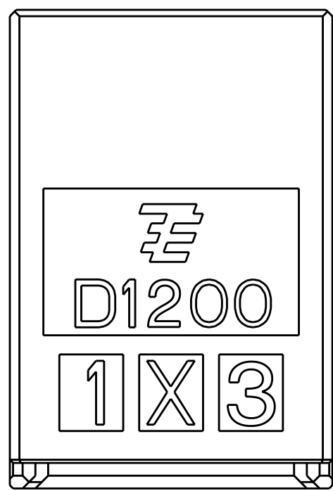
I-1827876-3 (6POS:X-KEY)
