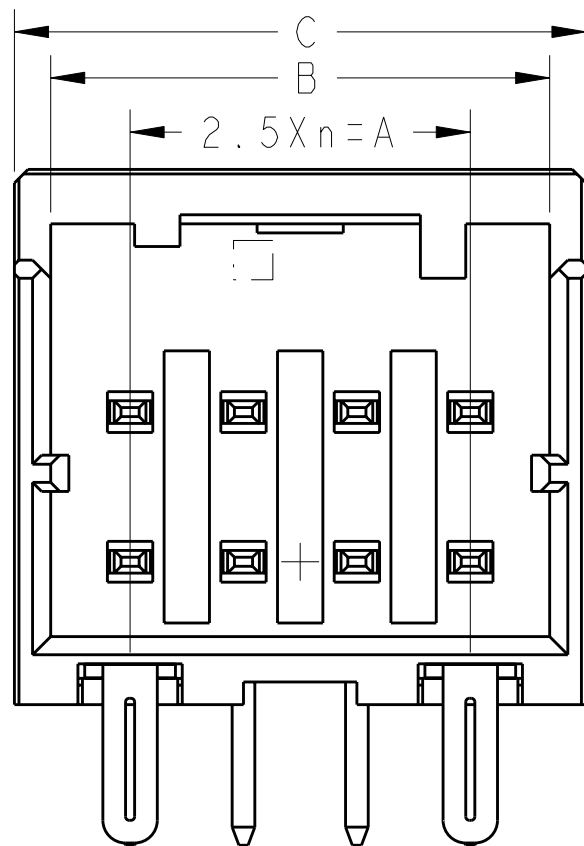
I-1827876-4 (8POS:X-KEY)
