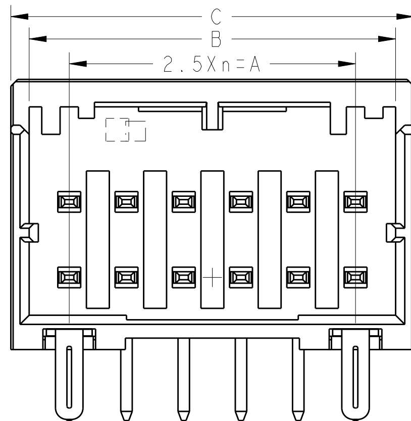
I-1827876-6 (12POS:X-KEY)
