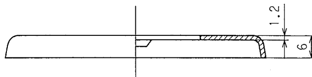
A-O-B断面図
