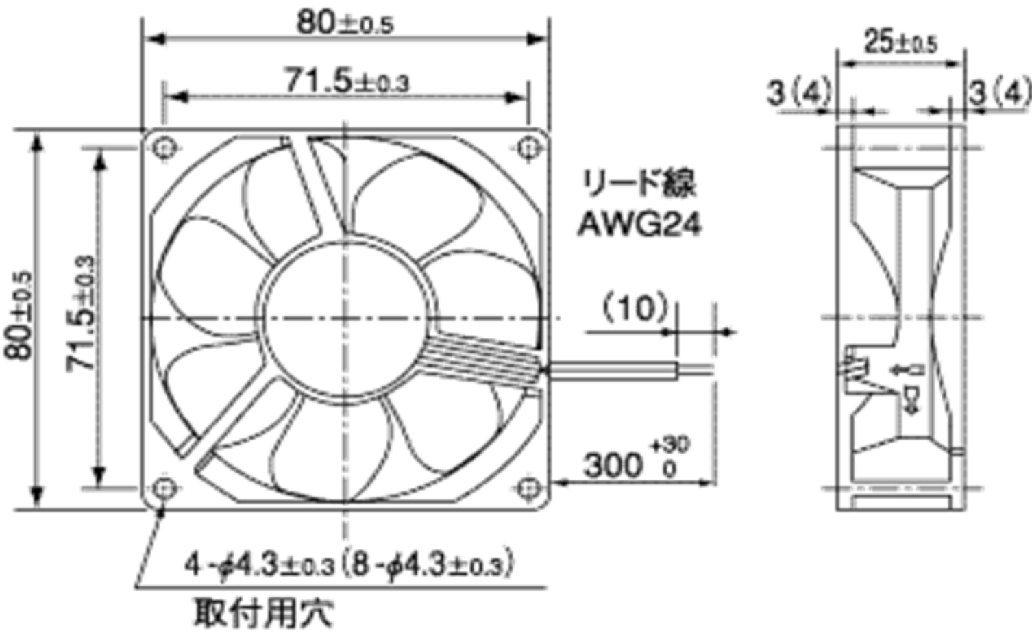
外形図
