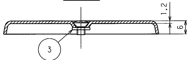
A-A'断面図
