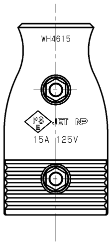
裏面刻印図
