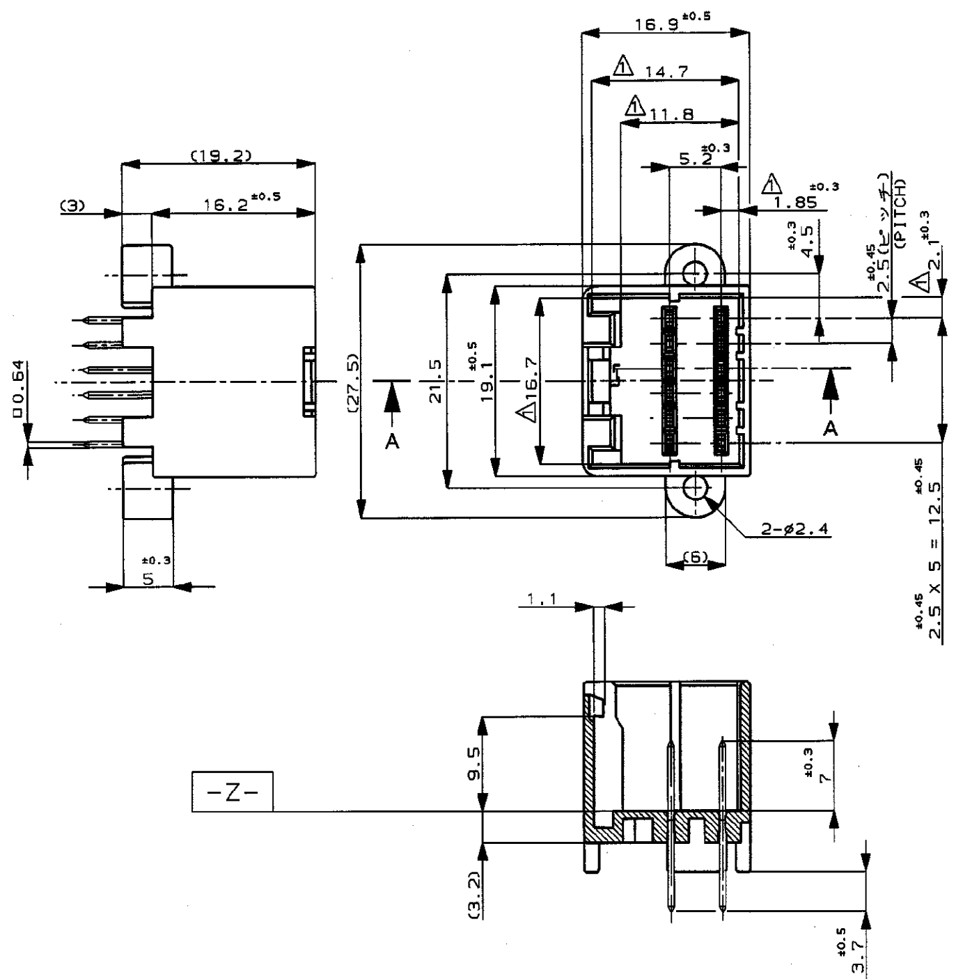
断面 A-A (SECT. A-A)
