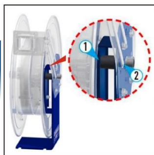
シャフトへの負荷を軽減する デュアルサポートシステム
