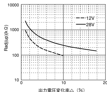
図2-5 \Delta(\%) 對外付け抵抗 (2)
