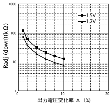
図2-6 △(%)對外付け抵抗 (3)
