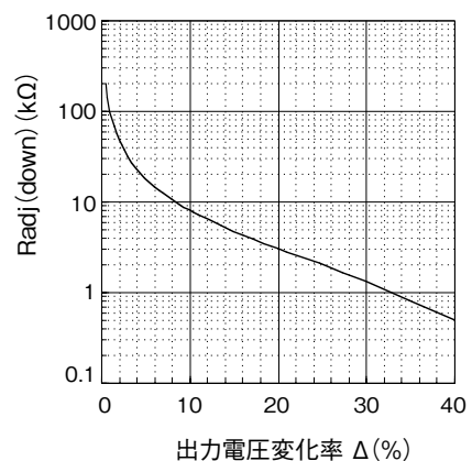
図2-3 \Delta (%) 対外付け抵抗 (1)
