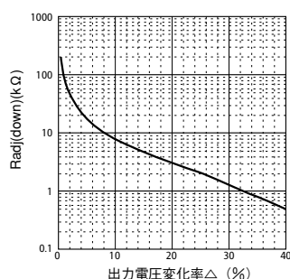
図2-3 \Delta(\%) 對外付け抵抗 (1)
