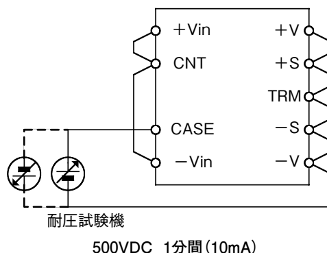
図19-2 出カーベースプレート間耐電圧試験方法
