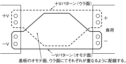
図9-3 両面基板を用いた負荷線パターンレイアウト例
