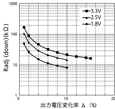
図2-5 △(%)對外付け抵抗 (2)
