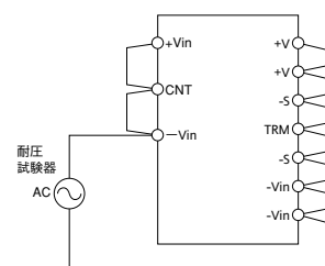
図19-1 入カ-出力間耐電圧試験方法
