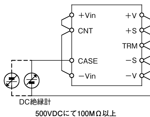
図20-1 絶縁抵抗試験方法
