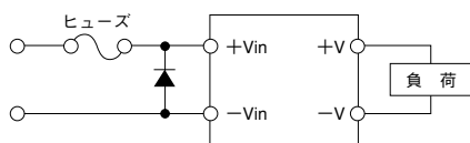
図1-5 入力逆接続保護
