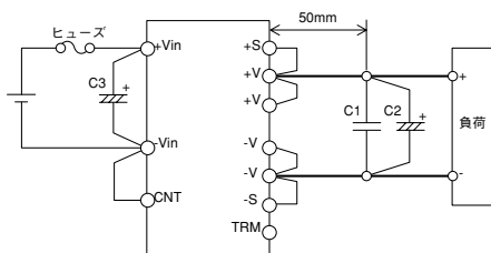
図1-2 基本的な接続
