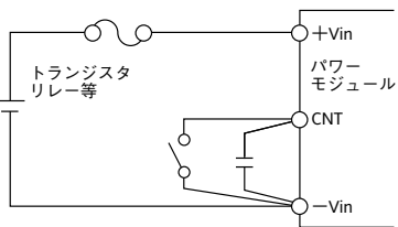
図10-1 CNT接続例 (1)
