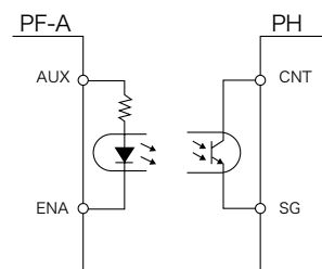
図16-1 PHシリーズとの接続例
