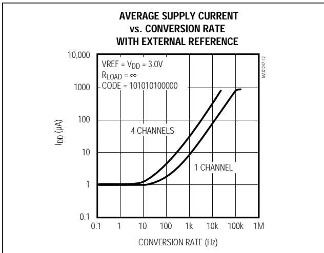
図12. 平均消費電流対変換レート(外部リファレンス)
