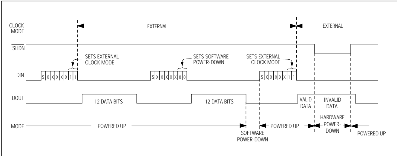
図11a. パワーダウンモードのタイミング図(外部クロック)
