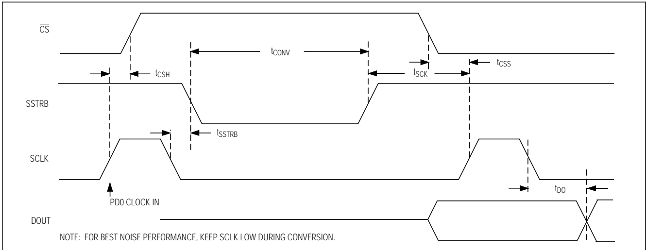
図9. 内部クロックモードでのSSTRBのタイミングの詳細
