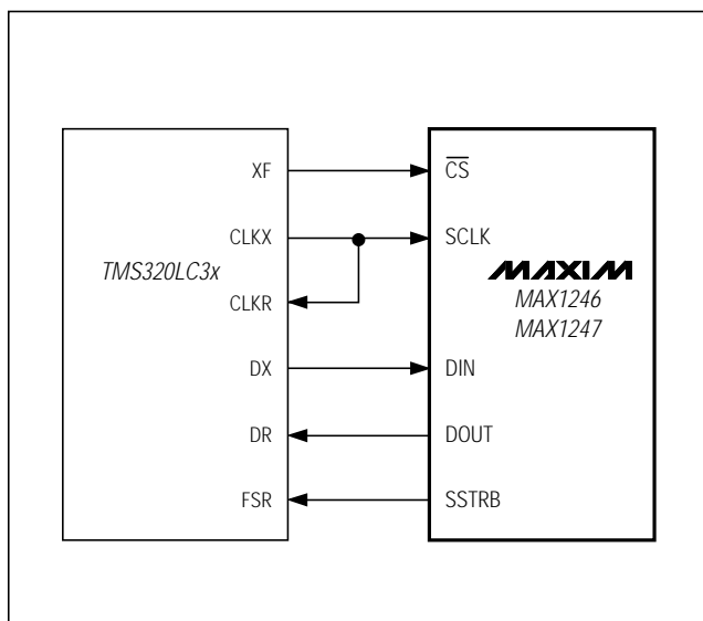
図20. MAX1246/MAX1247からTMS320への シリアルインタフェース
