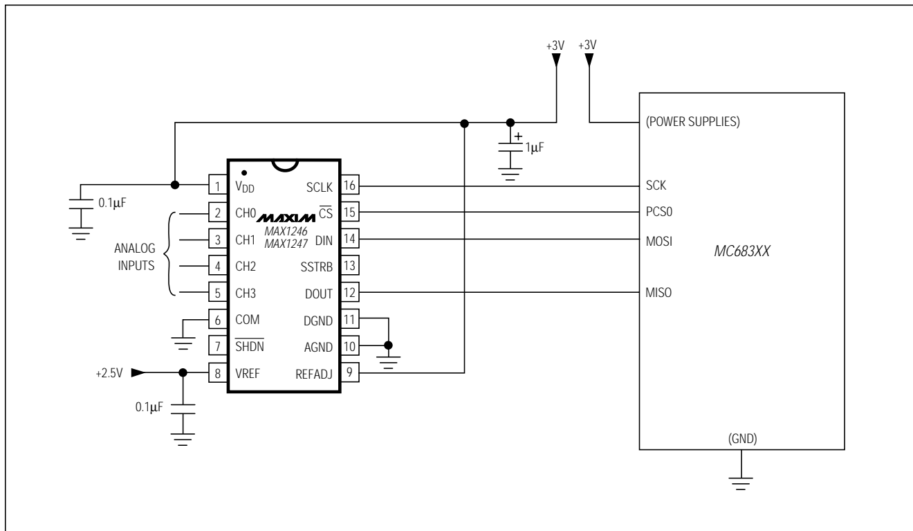
図19. MAX1246/MAX1247のQSPI接続図、外部リファレンス
