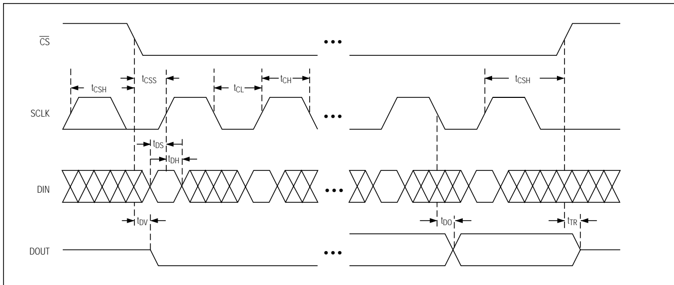
図6. シリアルインターフェースのタイミングの詳細
