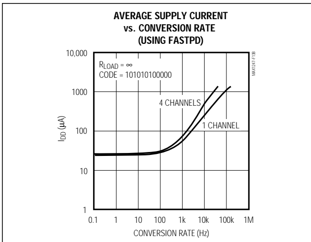
図13b. MAX1246の消費電流対変換レート(FASTPD)
