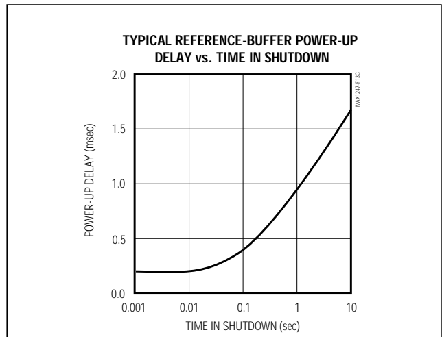
図13c. 標準リファレンスバッファパワーアップディレイ対シャットダウン時間
