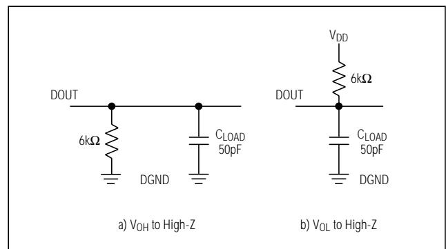
図2. ディセーブル時間用の負荷回路
