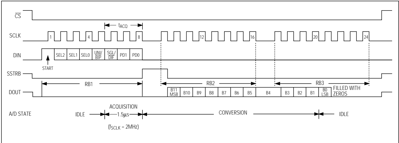
図5. 24クロック外部クロックモードの変換タイミング(MICROWIRE及びSPIコンパチブル、 f_{CLK} 2MHzでQSPIコンパチブル)
