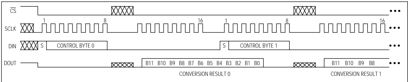
図10b. 外部クロックモード、16クロック/変換のタイミング
