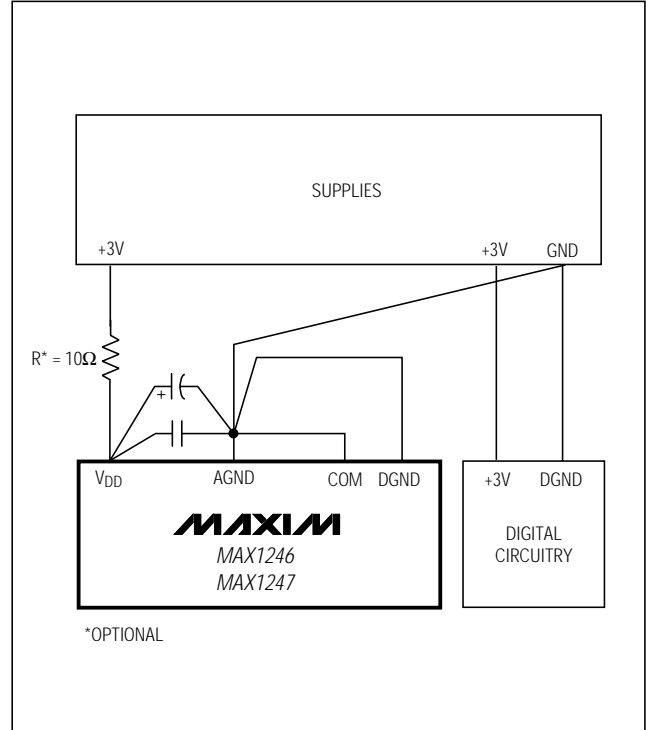
図18. 電源グランド接続図
