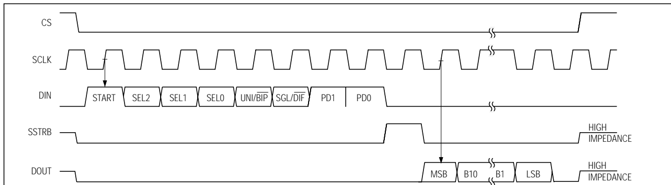
図21. TMS320のシリアルインタフェースタイミング図
