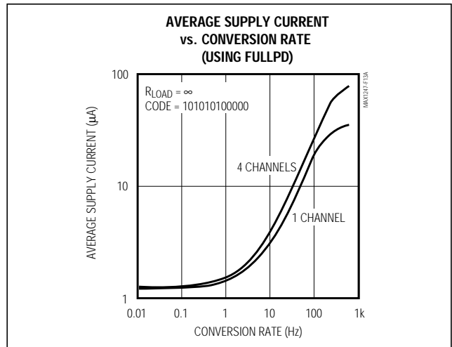
図13a. MAX1246の消費電流対変換レート(FULLPD)
