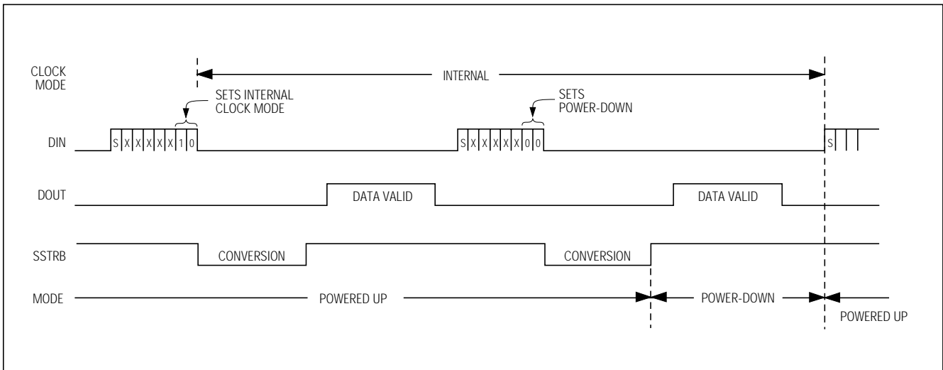
図11b. パワーダウンモードのタイミング図(内部クロック)
