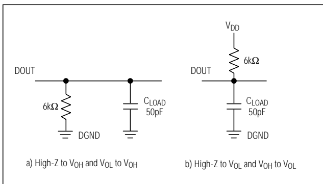
図1. イネーブル時間用の負荷回路
