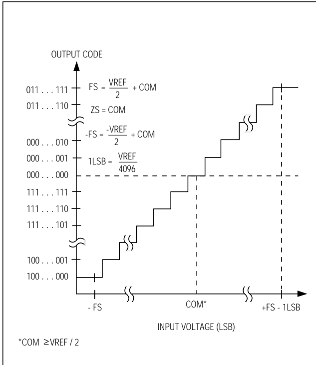
図17. バイポーラの伝達関数、フルスケール(FS) = V_{REF}/2 + COM 、ゼロスケール(ZS) = COM
