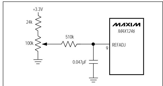
図15. MAX1246リファレンス調節回路
