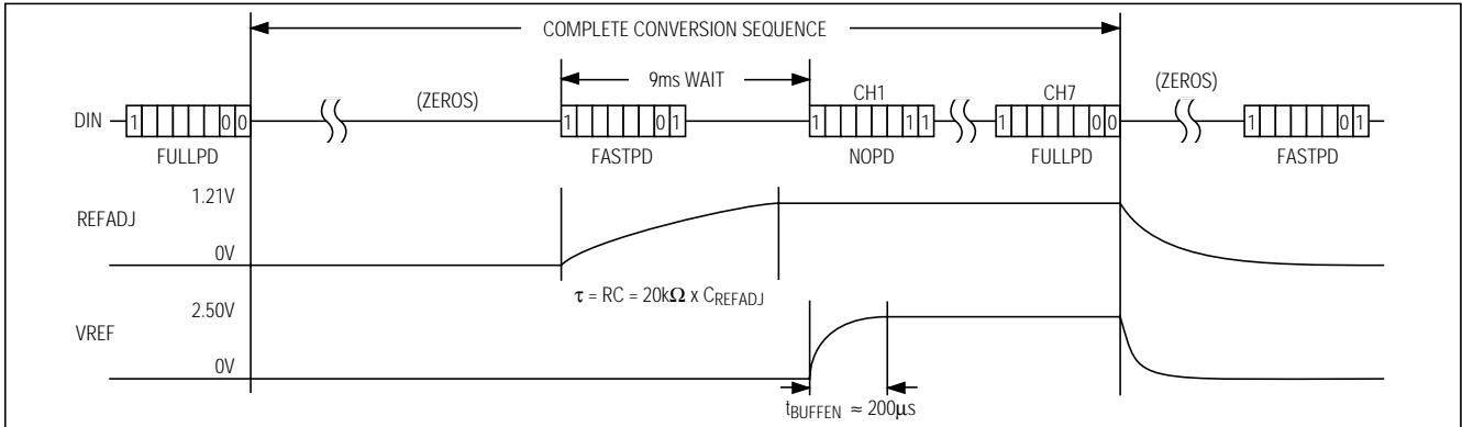
図14. MAX1246のFULLPD/FASTPDパワーアップシーケンス
