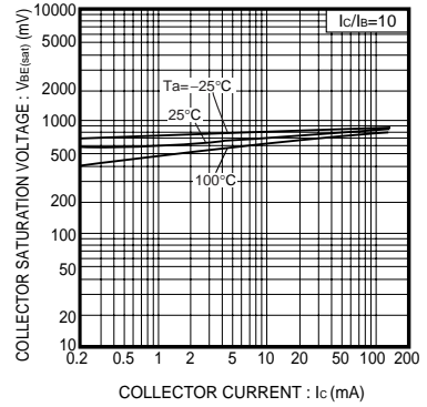
Fig.9 ベース・エミッタ間飽和電圧 -コレクタ電流特性 (II)
