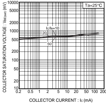
Fig.8 ベース・エミッタ間飽和電圧 -コレクタ電流特性 (I)
