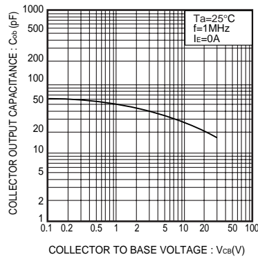
Fig.11 コレクタ出力容量 -コレクタ・ベース間電圧特性
