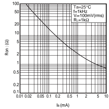
Fig.12 出力オン抵抗-ベース電流特性
