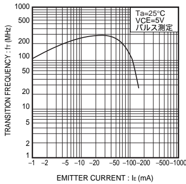
Fig.10 利得帯域幅積-エミッタ電流特性
