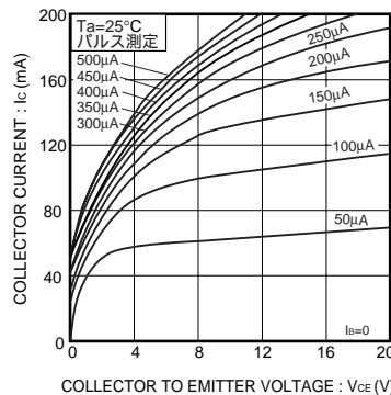
Fig.2 エミッタ接地出力静特性 (II)
