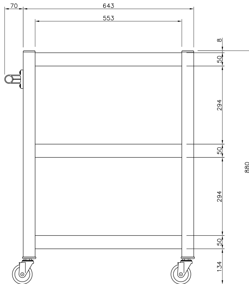
組み付け寸法例
