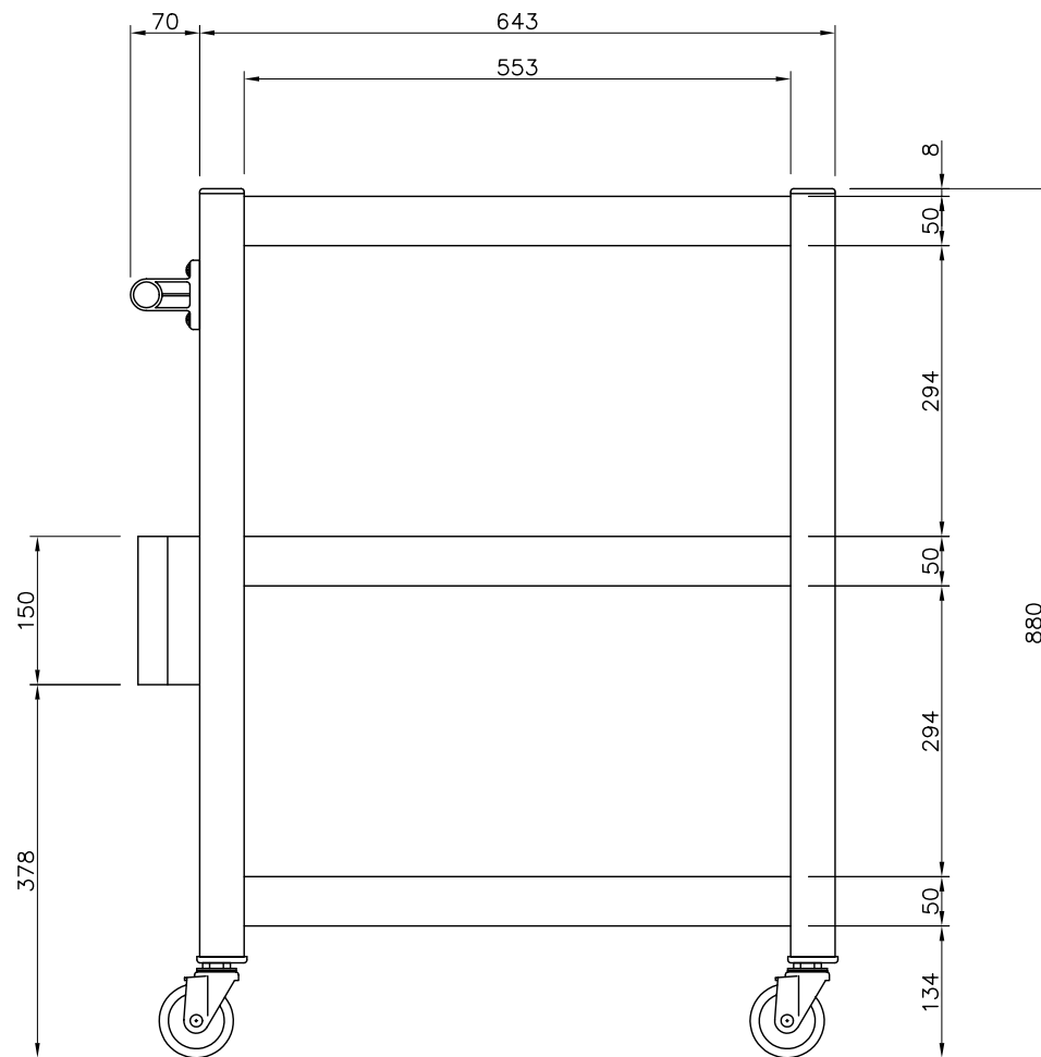
組み付け寸法例
