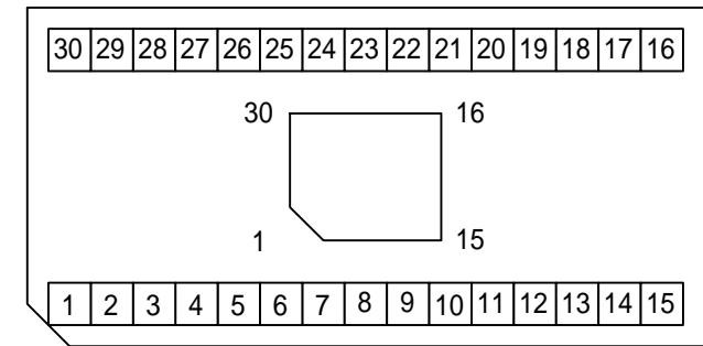
ピン番号図 (上面図)
