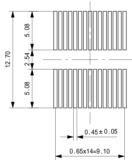
パッド部上面図 Scale4:1
