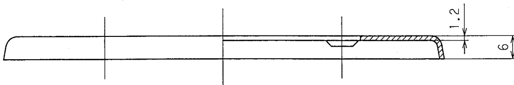
A-O-B断面図
