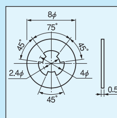
品番 2.6MT-W (M2.6用)
