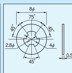
品番 3MT-W (M3用)
