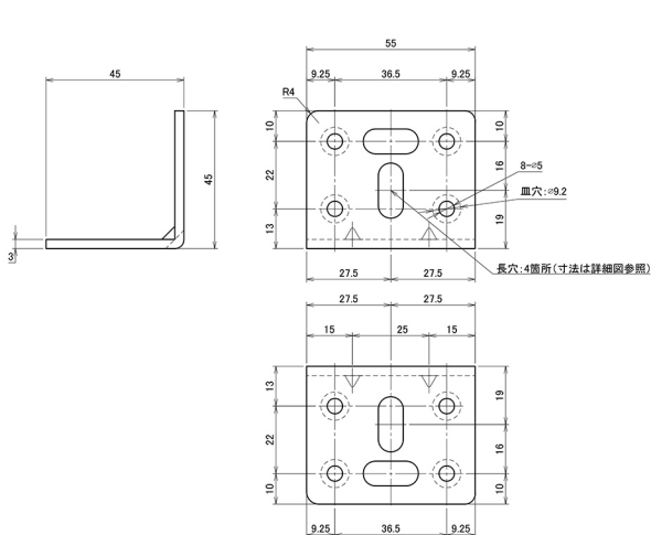
長穴詳細図 S:1/1
