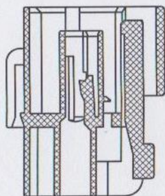
剖面 A-A
