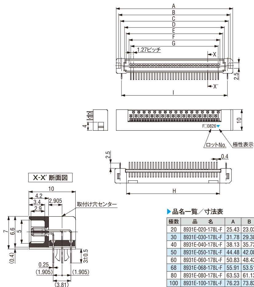
▶ 参考基板設計要領(コネクタ搭載面)
