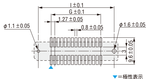
▶ 参考基板設計要領(コネクタ搭載面)
