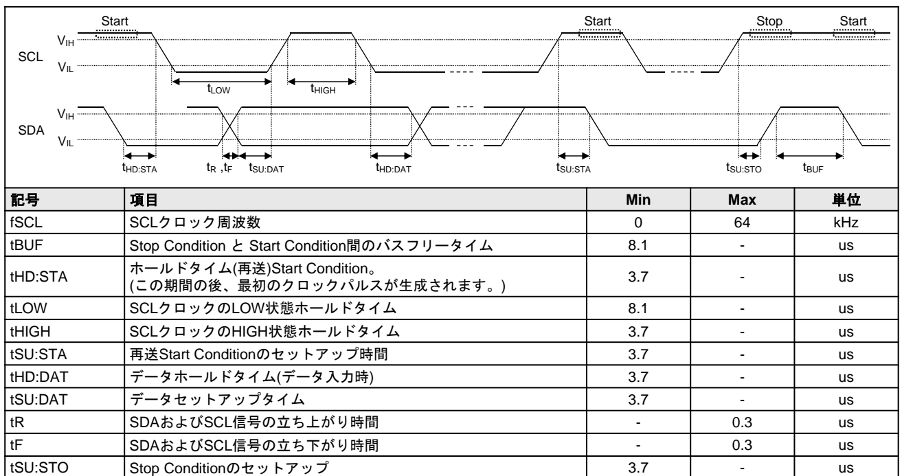
図8.8.2 2線シリアル通信 SCL, SDA タイミング仕様(参考)
