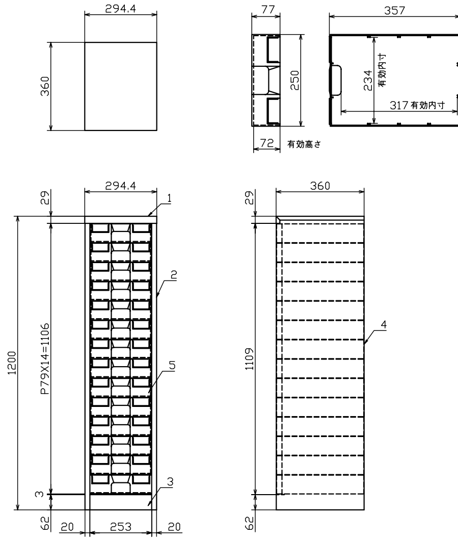
引出詳細図
