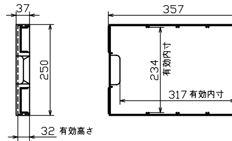
引出詳細図
