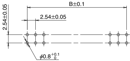
◆推奨基板寸法図
