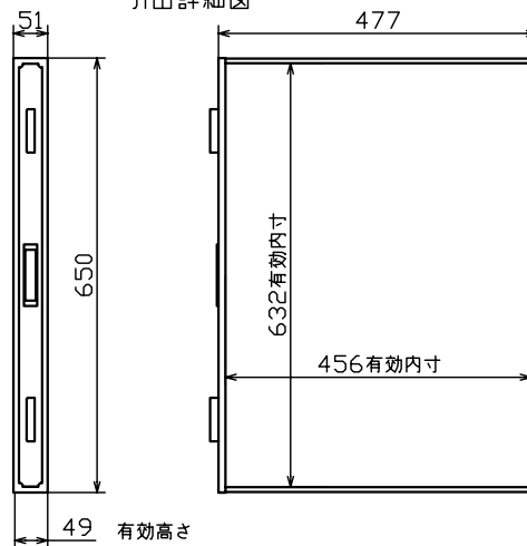
引出詳細図
