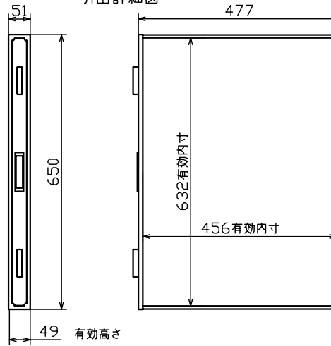
引出詳細図
