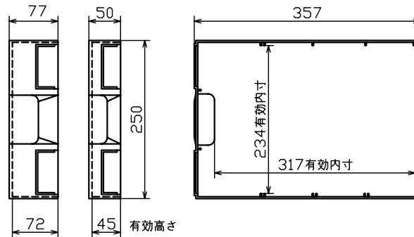
引出詳細図
