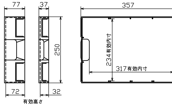
引出詳細図
