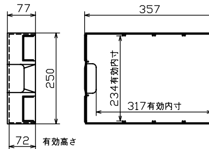
引出詳細図
