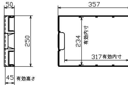
引出詳細図
