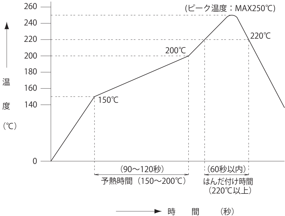
推奨温度プロファイル
