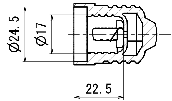
A-A ( 1 : 1 )
