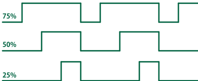
図16 デューティ比の変更
