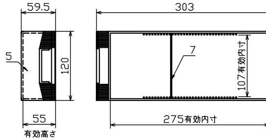
引出詳細図
