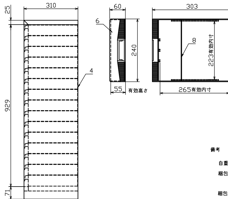
引出詳細図
