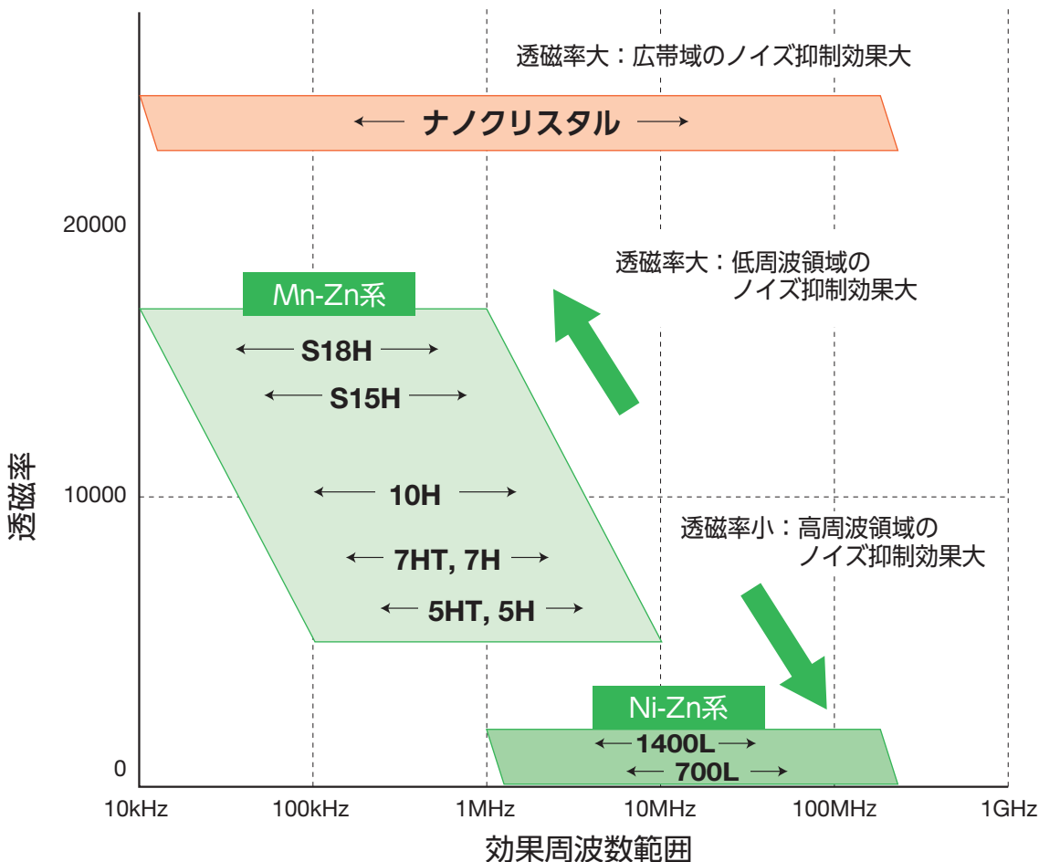
図2 透磁率による効果周波数範囲の関係
