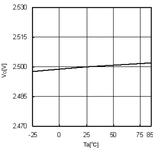
Fig.10 T_a-V_O ( I_o=0A )
