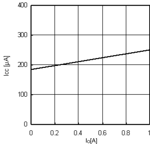
Fig.32 I_o - I_{cc}
