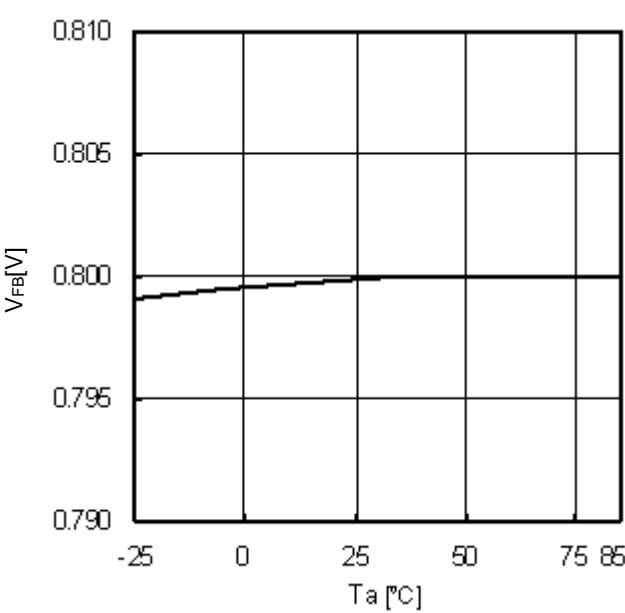
Fig.9 T_a-V_{FB}
