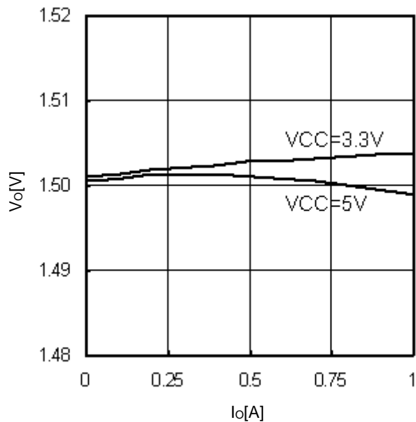
Fig.16 Io-Vo (Vo=1.5V)
