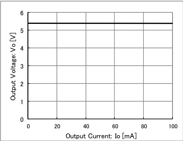
Figure 9. Io - Vo
