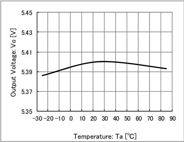
Figure 6. Ta - Vo (Io = 0mA)
