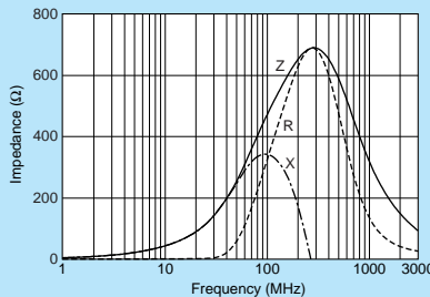
BLA2ABD471SN4
