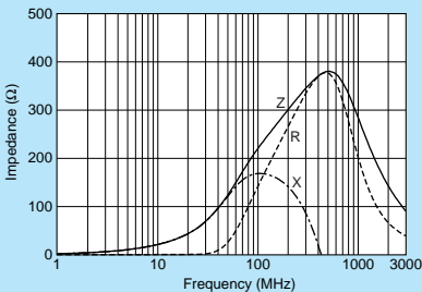
BLA2ABD221SN4
