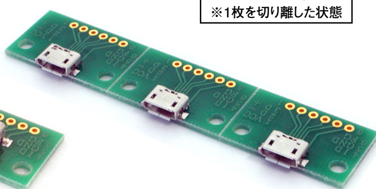
CK-37 (Micro-USB Micro-ABタイプコネクタ実装済み)
