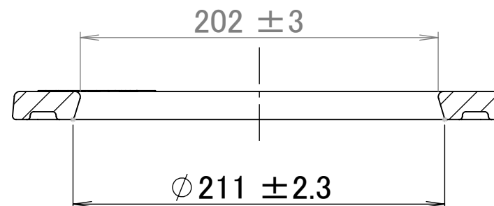
断面図 a-a
