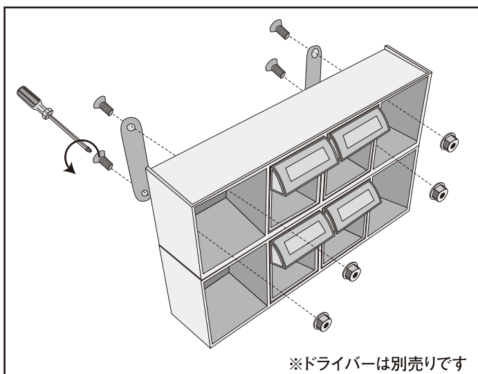
②上図のように取付けます ※本体の向きに気を付けてください。
