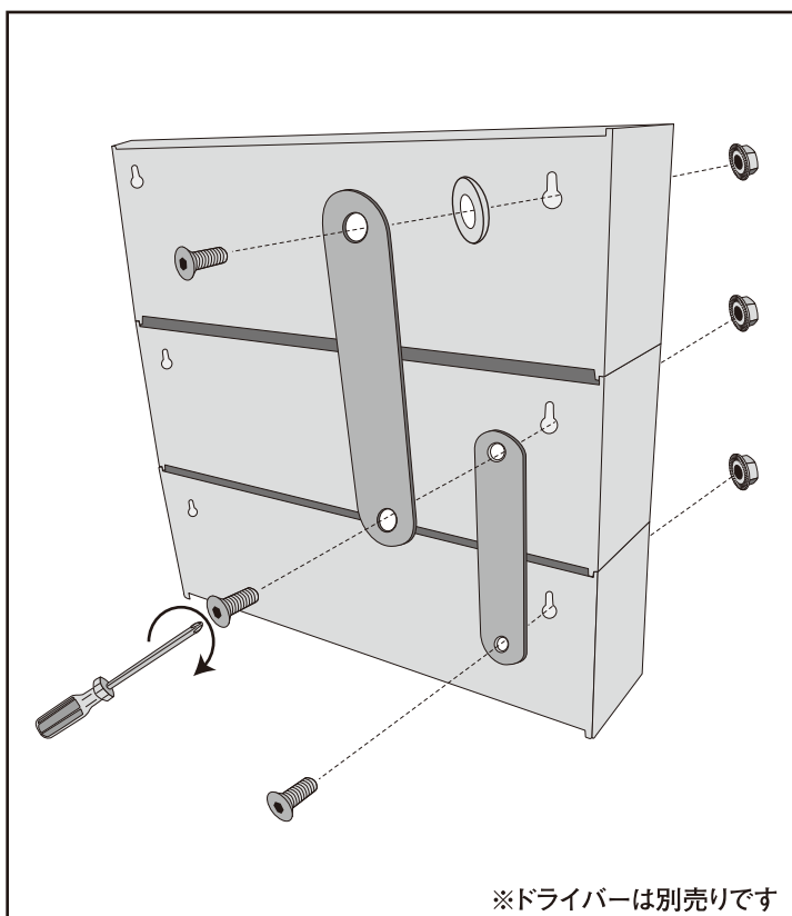
※三段にする場合は上図のように取り付けてください。
