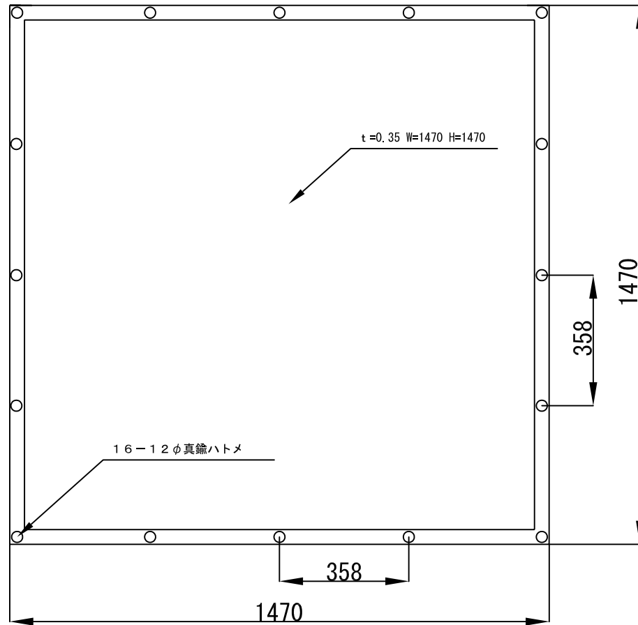
平 面 図
