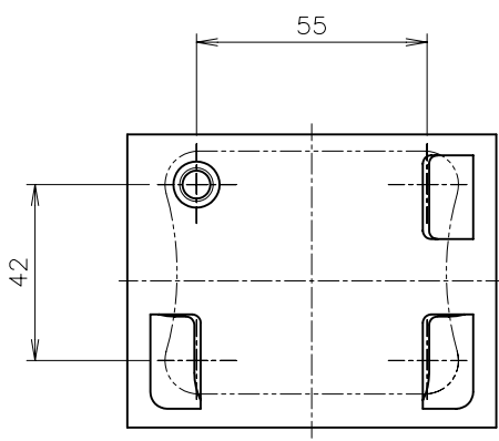
取付部詳細図 (S=1:2)
