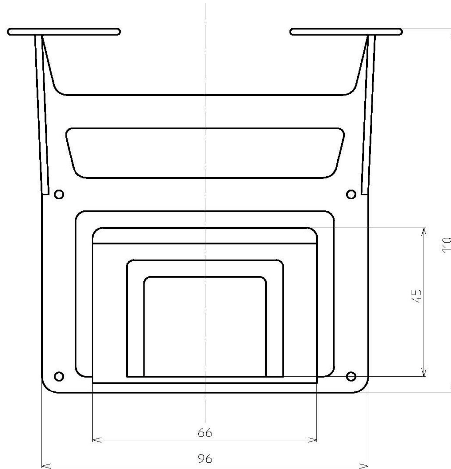
正面図
