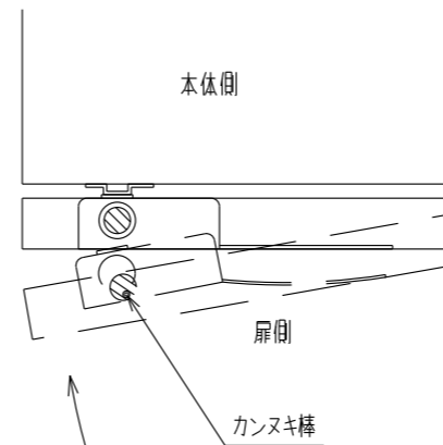
B-B断面図(S-1/5)
